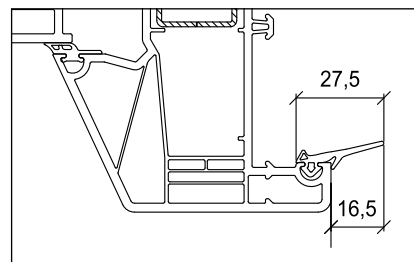
i-Kozijn NL afdichting
