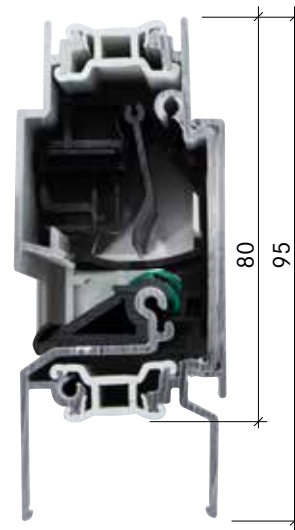
DucoFlat 12 'ZR' Voor glasdiktes: 28/32 mm
